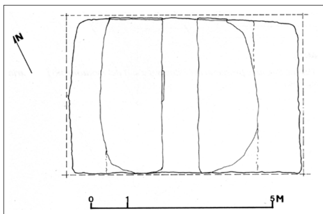
Fig. 132. Urbisaglia, rilievo planimetrico del monumento funerario 055.015 (da CATANI 1990, p. 162, fig. 15).
