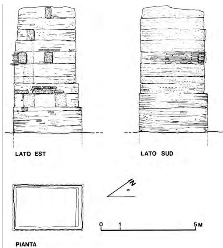
Fig. 142. rilievo del secondo monumento funerario nel sito 055.066 (da CATANI 1990, p. 154, fig. 4).
