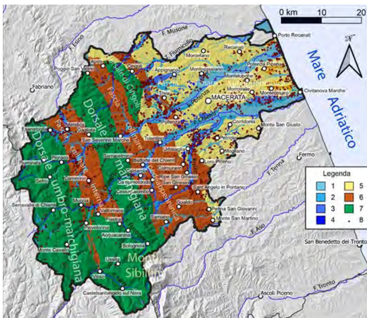
Fig. 6. Carta geologica schematica della Provincia di Macerata. 1 – depositi alluvionali del 4° ordine; 2 – depositi alluvionali del 3° ordine; 3 – depositi alluvionali del 2° ordine; 4 – depositi alluvionali del 1° ordine; 5 – successione sedimentaria umbro-marchigiana plio-pleistocenica; 6 – successione sedimentaria umbro-marchigiana miocenica; 7 – successione sedimentaria umbro-marchigiana giurassico-miocenica; 8 - puntini rosso/neri i siti archeologici (elaborazione degli AA.).
