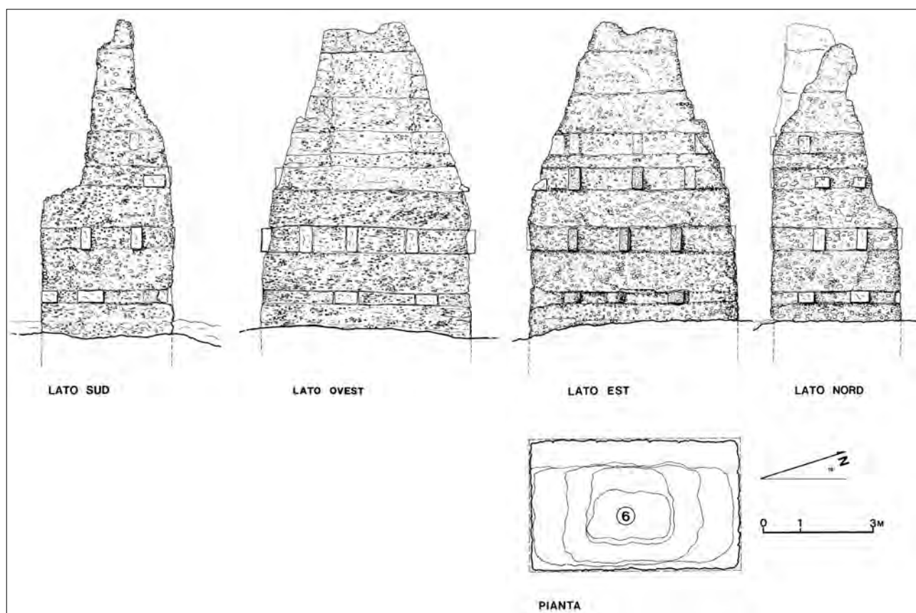
Fig. 130. Urbisaglia, località Abbadia. Rilievo di uno dei due monumenti funerari (da CATANI 1990, pp. 156-157, figg. 6, 7.
