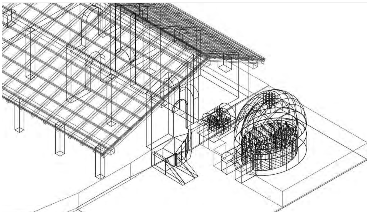
Fig. 108. San Severino Marche, località Pieve. Complesso artigianale presso il tratto ovest delle fortificazioni di Septempeda, ipotesi di ricostruzione delle volumetrie (elaborazione D. Sforzini).
