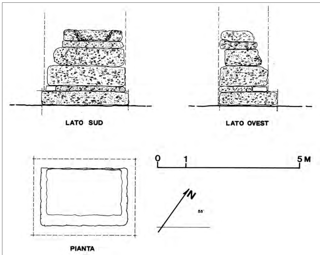
Fig. 151. Urbisaglia, C.da Fiastra. Monumento funerario nel settore della necropoli orientale della città romana, rilievo (da CATANI 1990, p. 160, fig. 13).
