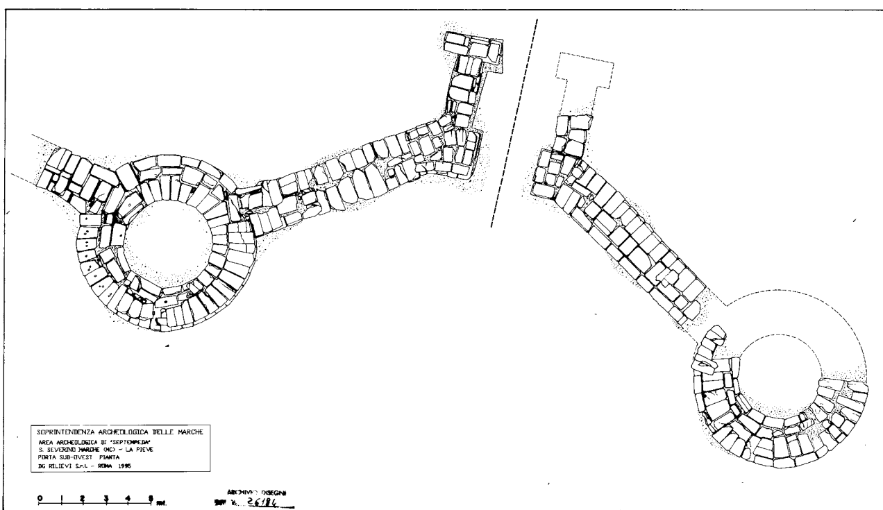
Fig. 102. San Severino Marche, località Pieve. Rilievo delle strutture pertinenti alla porta sud-occidentale della città romana di Septempeda (SABAP AP-FM-MC, Archivio Disegni, nn. 26183, 26184).
